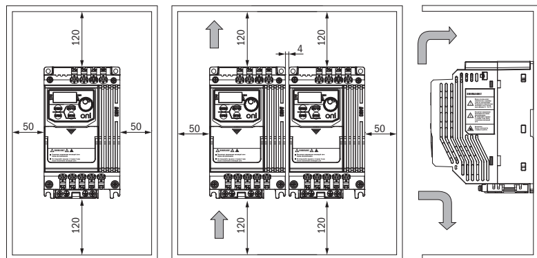
Рисунок 3.2. Установка преобразователей
