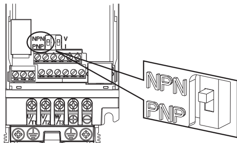
Рисунок 4.4.1. DIP-переключатель режимов NPN/PNP
